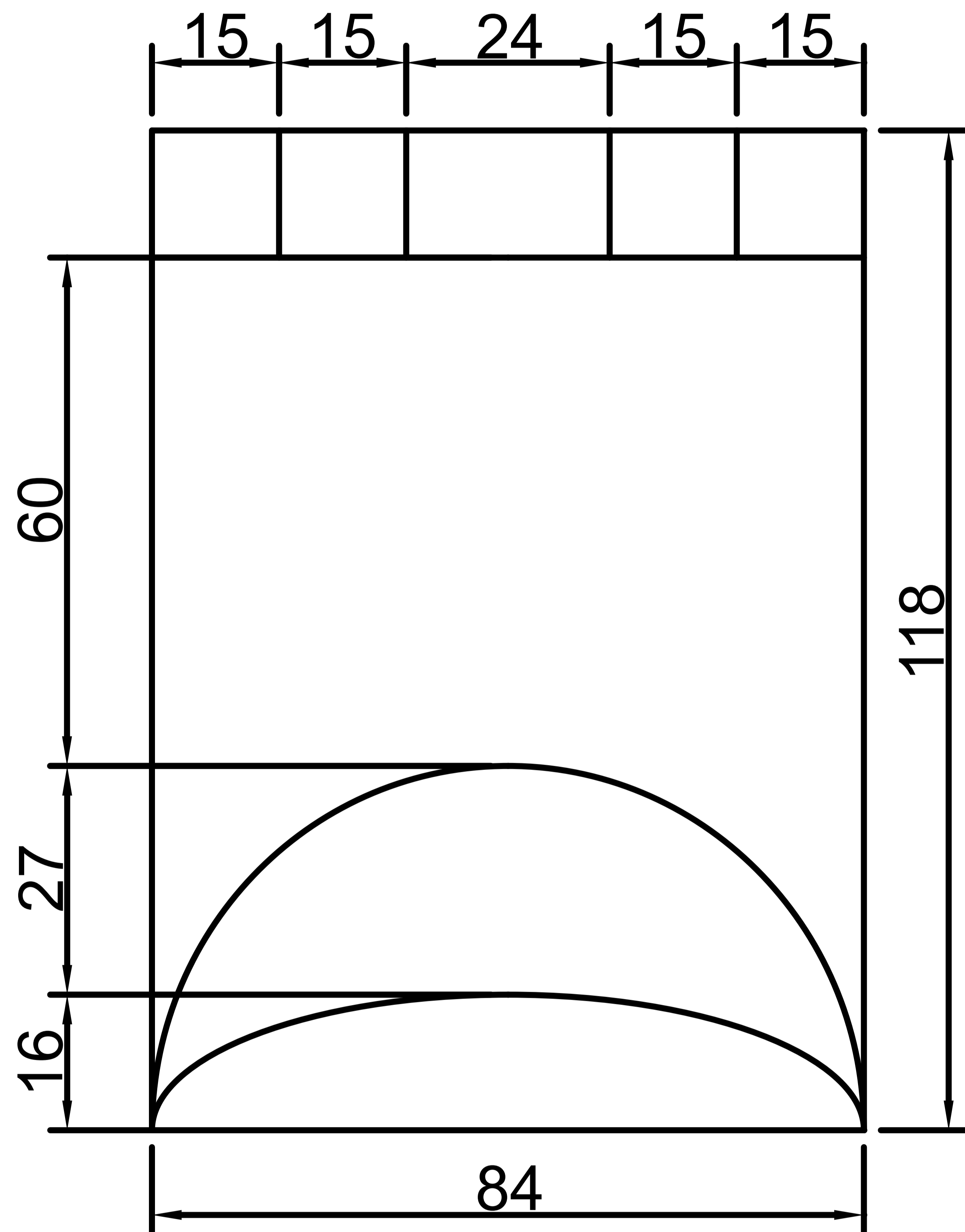
三分勇士尺寸
